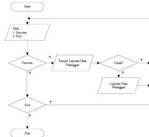
Gambar 13. Flowchart Laporan Data Pelanggan
