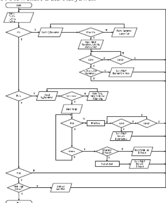
F. Flowchart Data Karyawan
