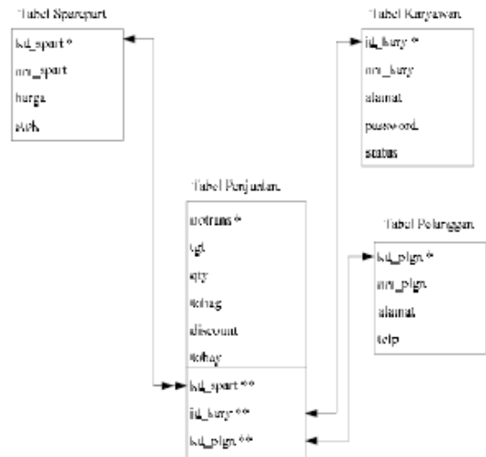
Gambar 3. Bentuk Normal Kedua
