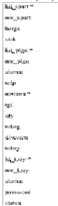
Gambar 2. Bentuk Normal Kesatu
